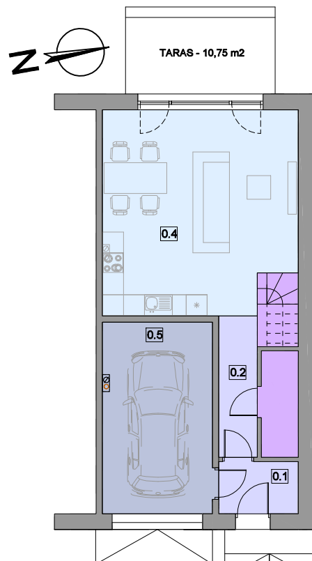
RZUT PARTERU - 59,50 m 2
