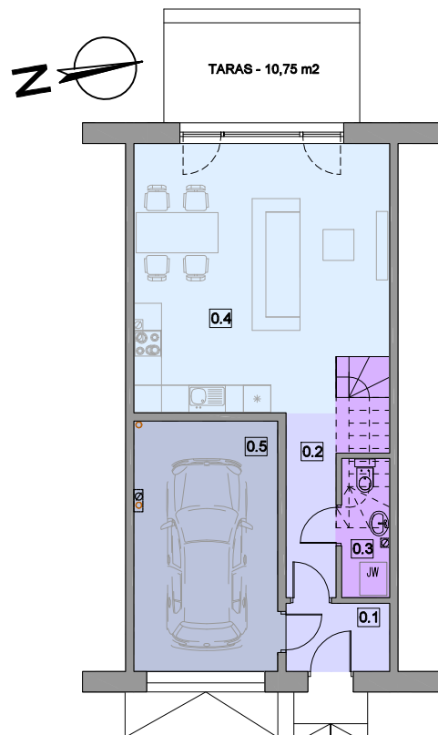
RZUT PARTERU - 59,50 m 2
